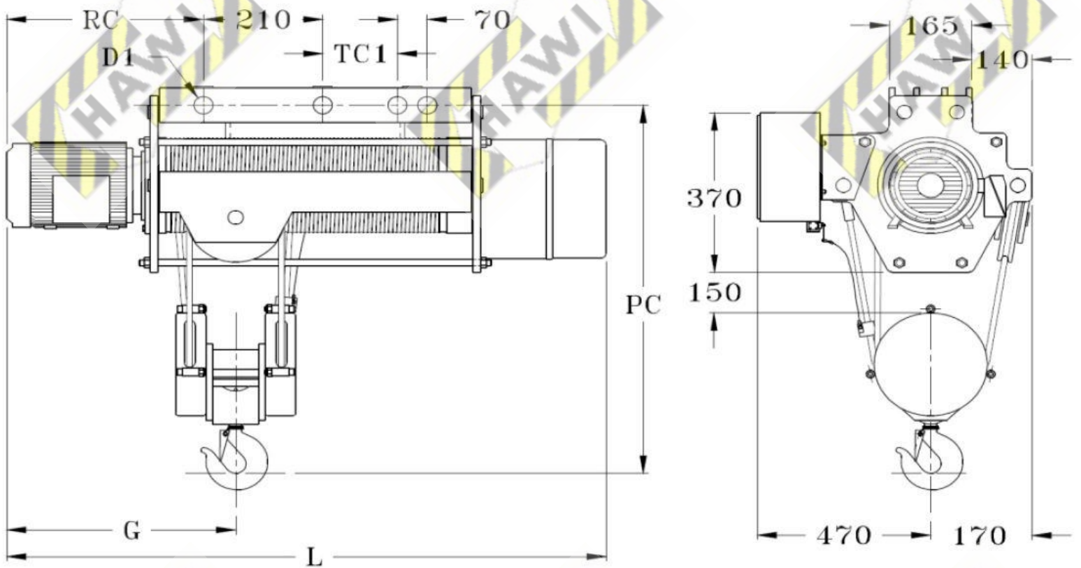
TIPO FIJO COLGANTE EXTENDIDO
