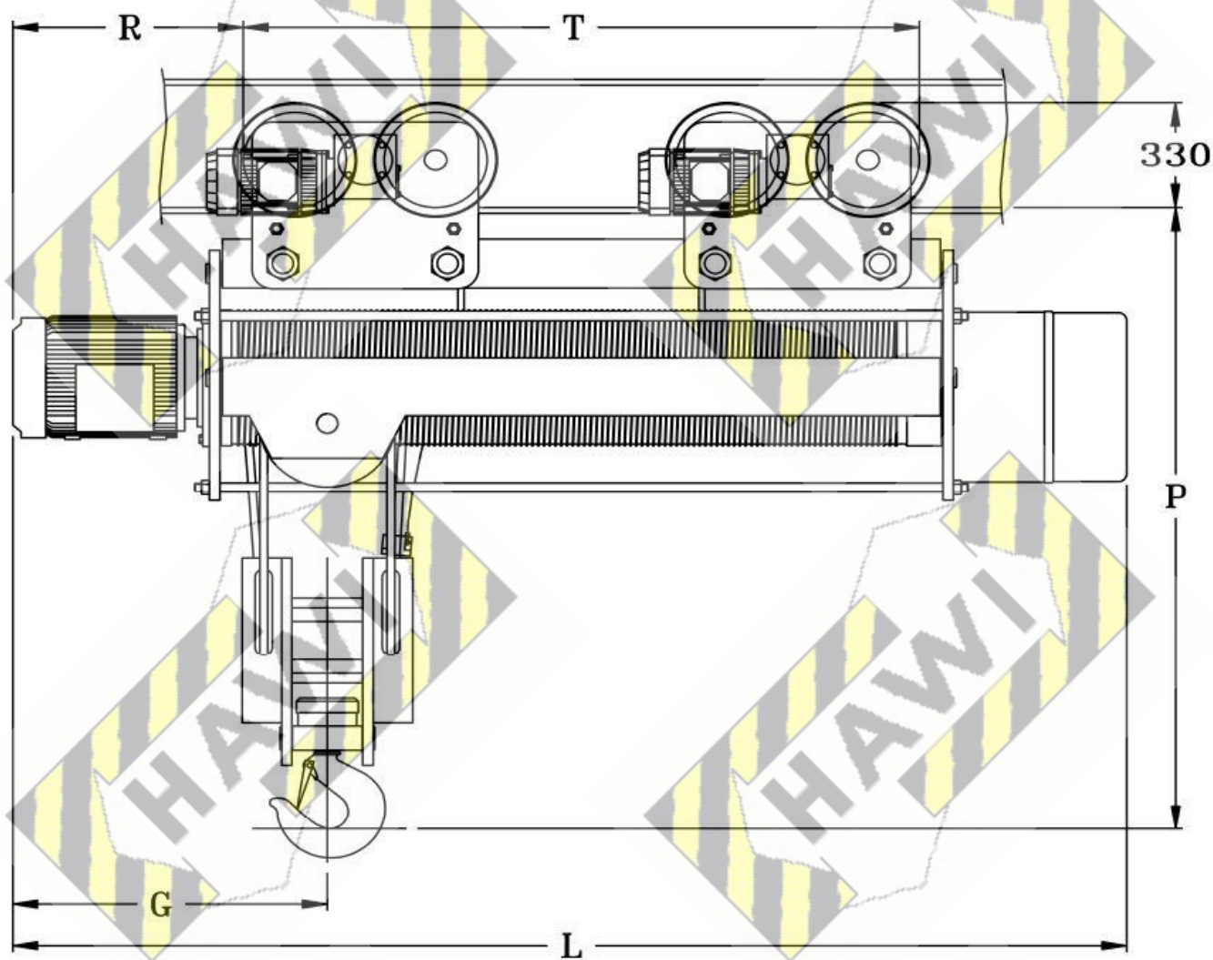
TIPO DOBLE CARRO MOTORIZADO
